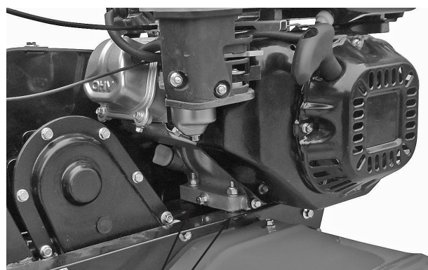
Figura 11 Dadi motore
