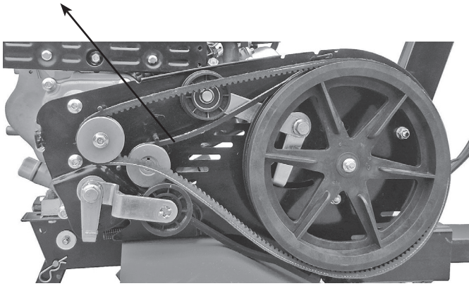
Figura 10 Porcas do motor
