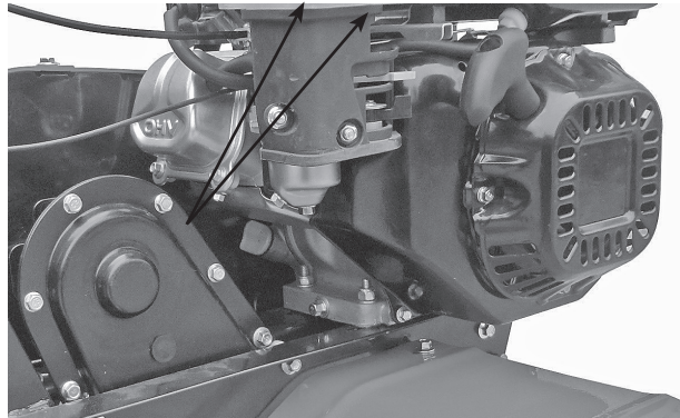
Figur 11 Motorrens monteringsbultar
