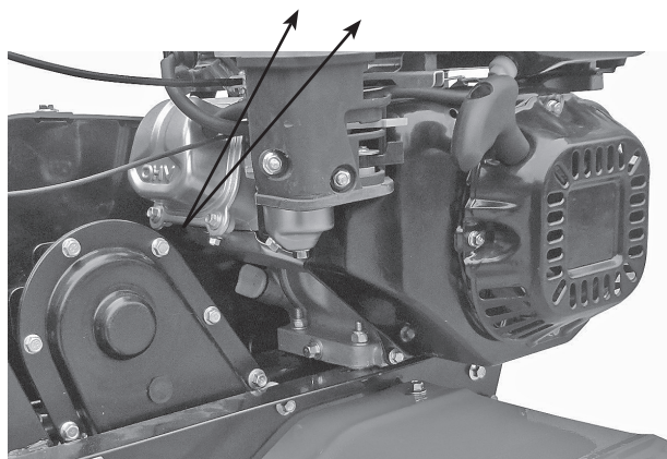
Фигура 11 Гайки на двигателя
