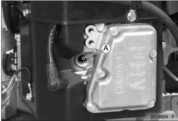
A. Orifício da vela de ignição
